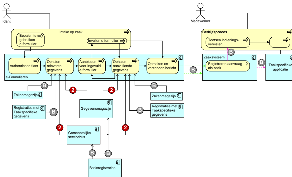
Figuur 6. Applicatiearchitectuur
