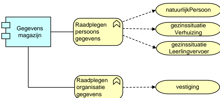
Figuur 4. Services met betrekking tot het gegevensmagazijn
