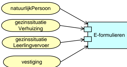
Figuur 3. De door de e-formulierenapplicatie gebruikte services
