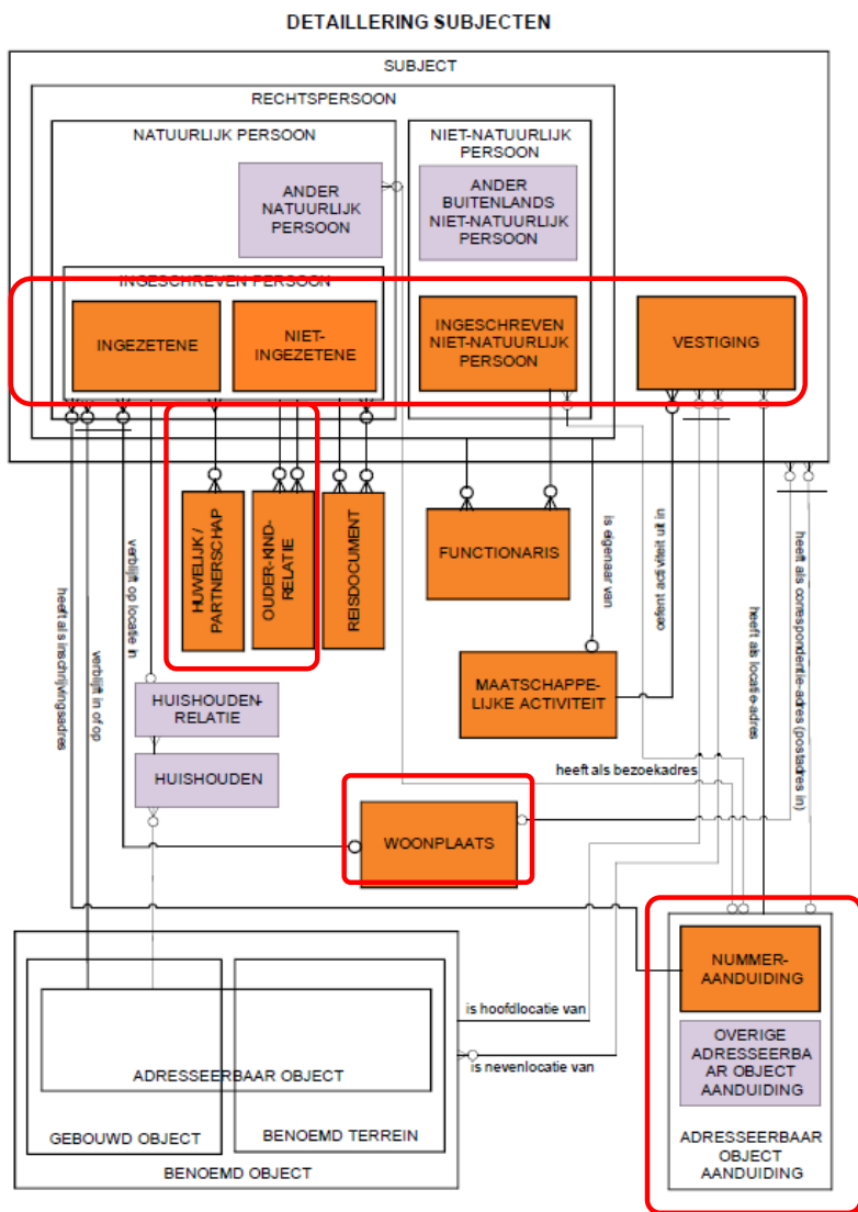
Figuur 9. Detaillering betrokken objecten uit RSGB
