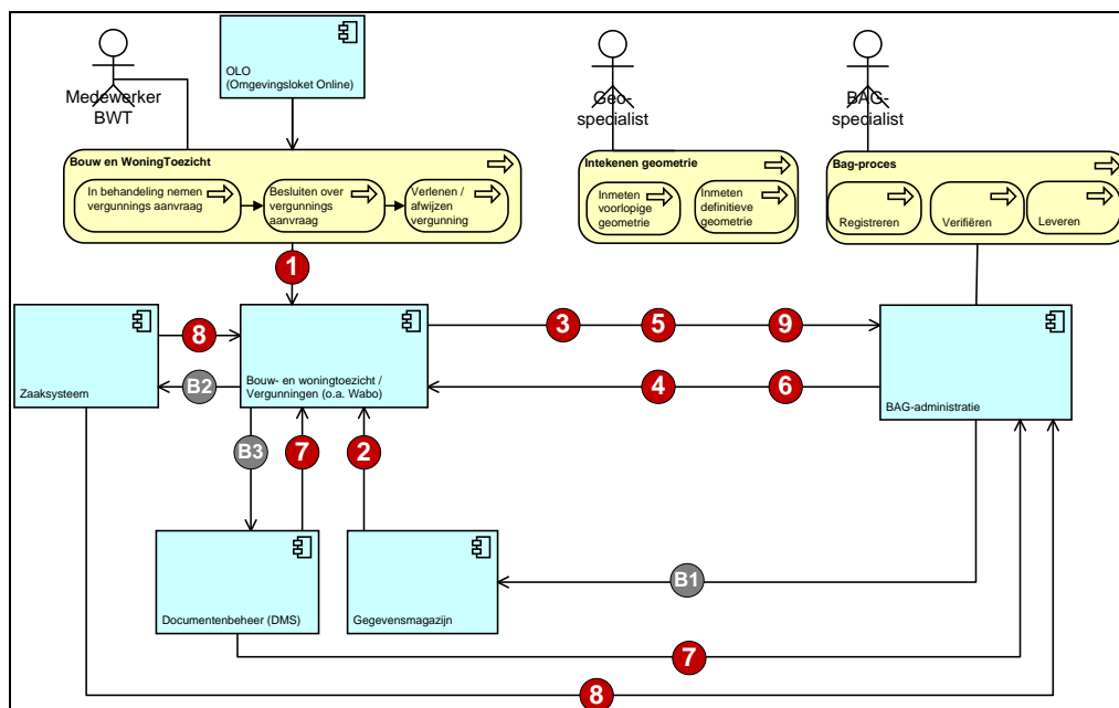
Figuur 2 De referentiearchitectuur
