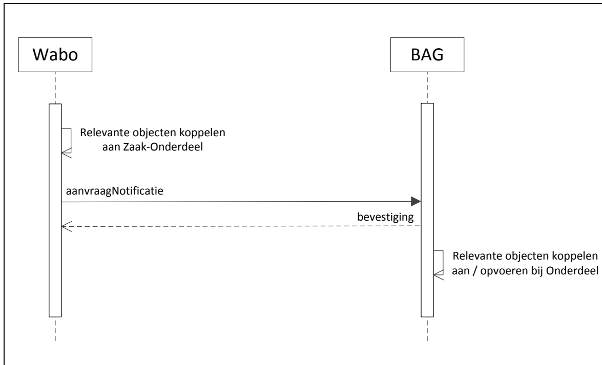
Figuur 6 Interactiemodel Aanvraagnotificatie
