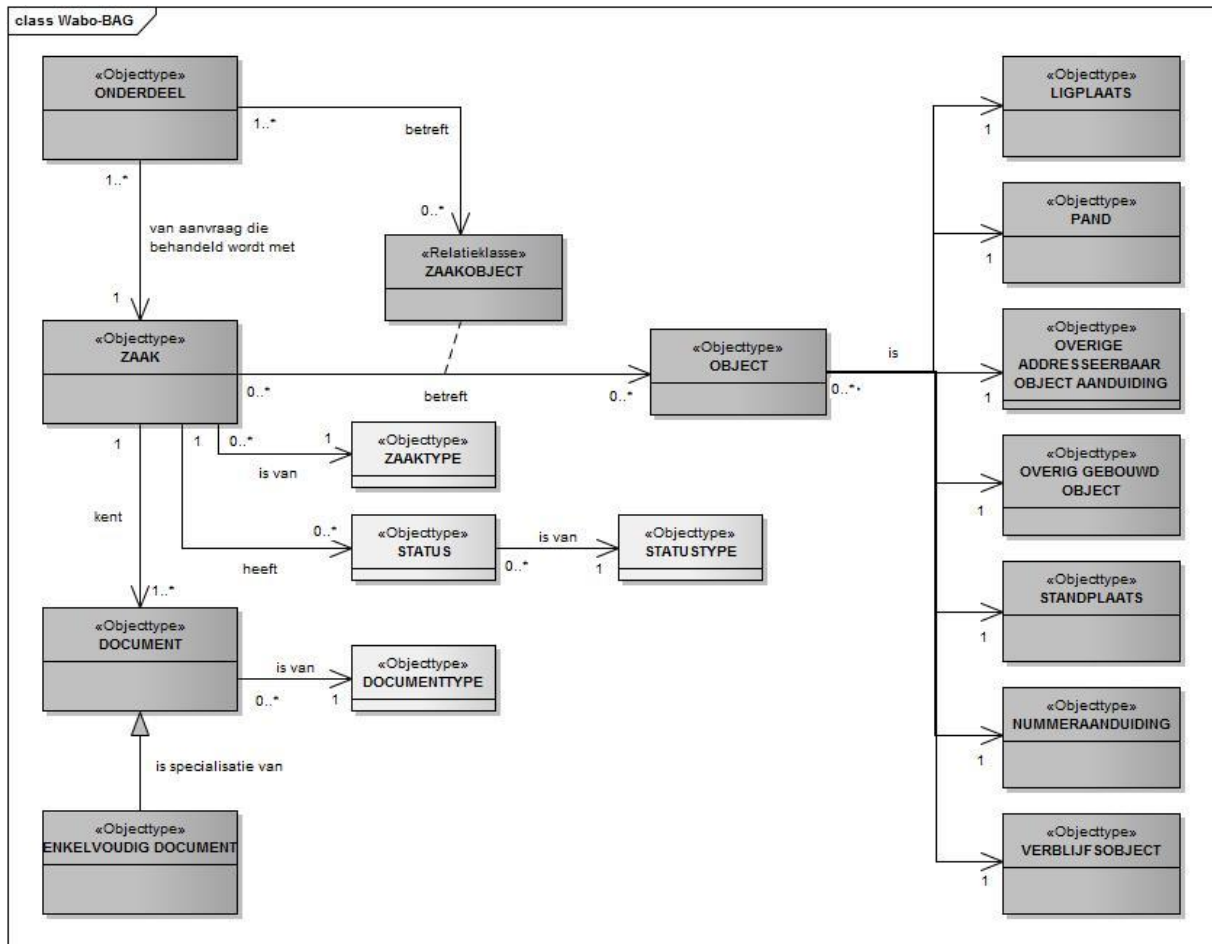
Figuur 3 Informatiemodel Wabo-BAG
