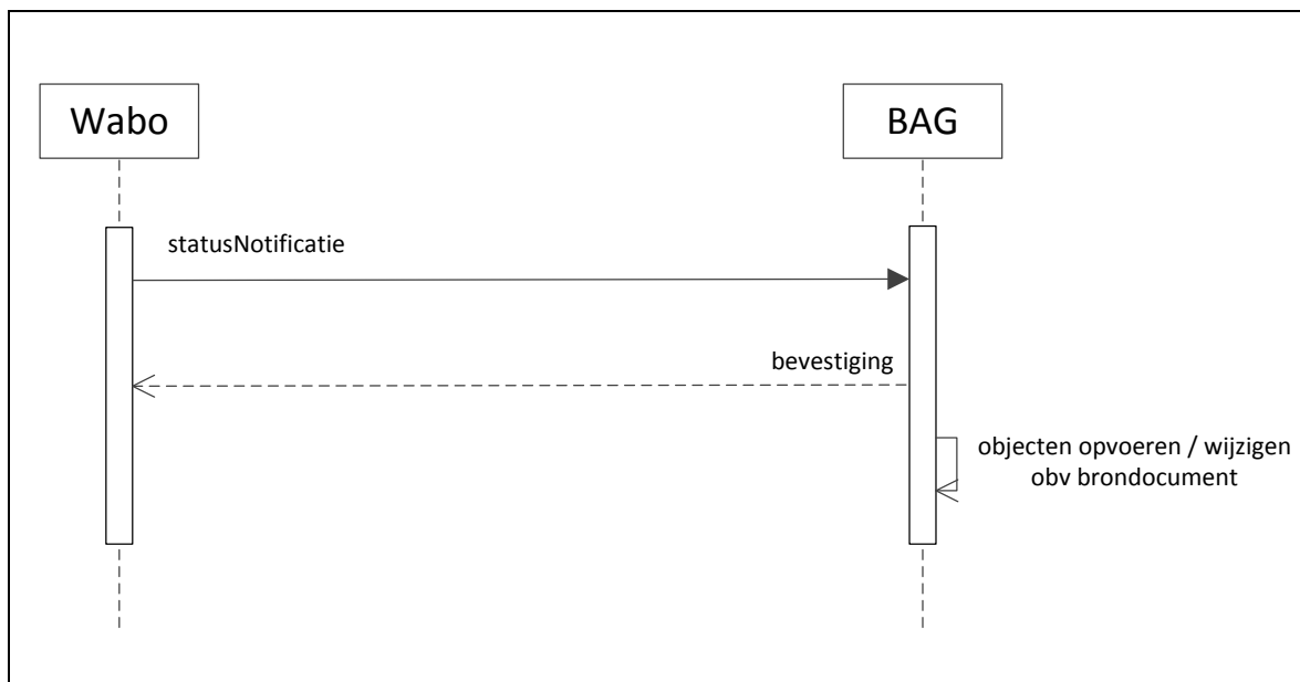
Figuur 8 Interactiemodel Statusnotificatie
