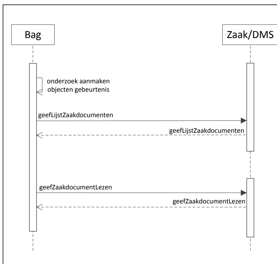
Figuur 11 Interactiemodel Opvragen zaakdocumenten
