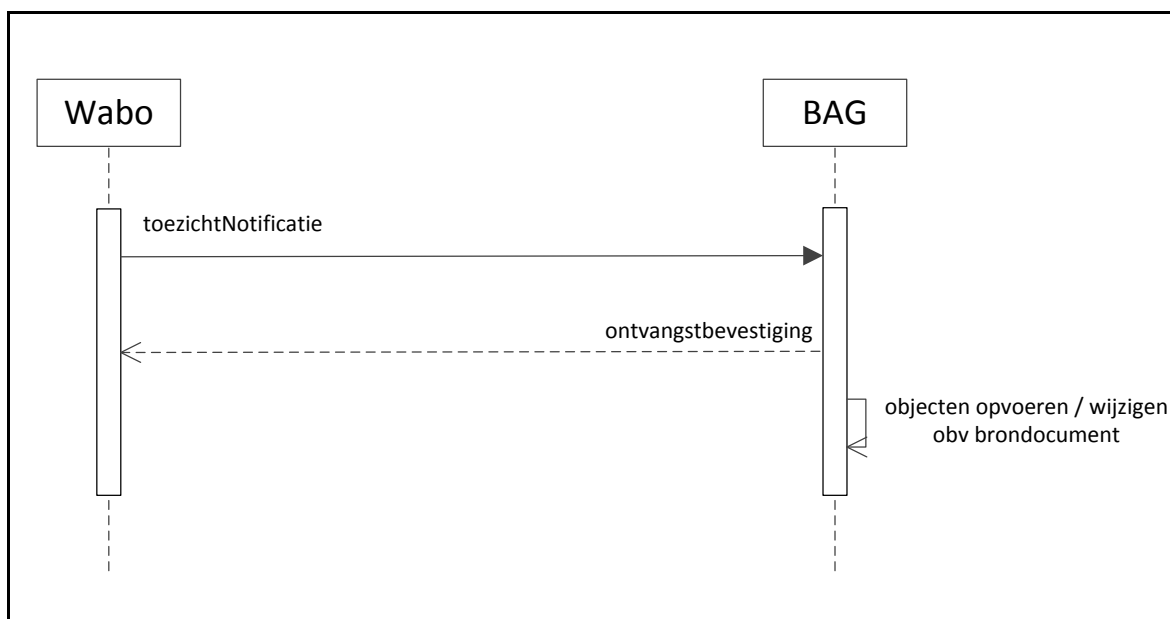
Figuur 9 Interactiemodel ToezichtNotificatie
