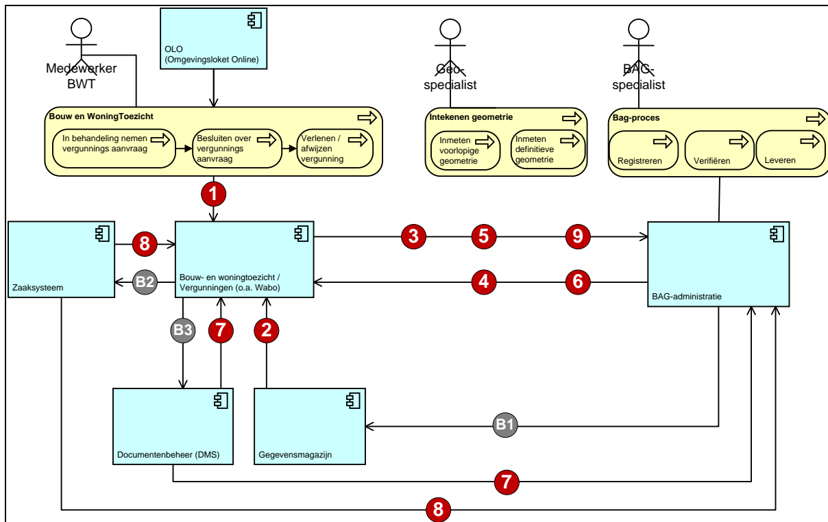
Figuur 2 De referentiearchitectuur
