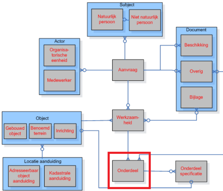
Figuur 12 Informatiemodel OLO (bron: functioneel ontwerp OLO)
