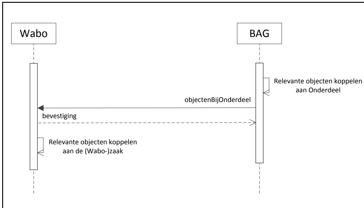
Figuur 7 Interactiemodel Objectenbijonderdeel
