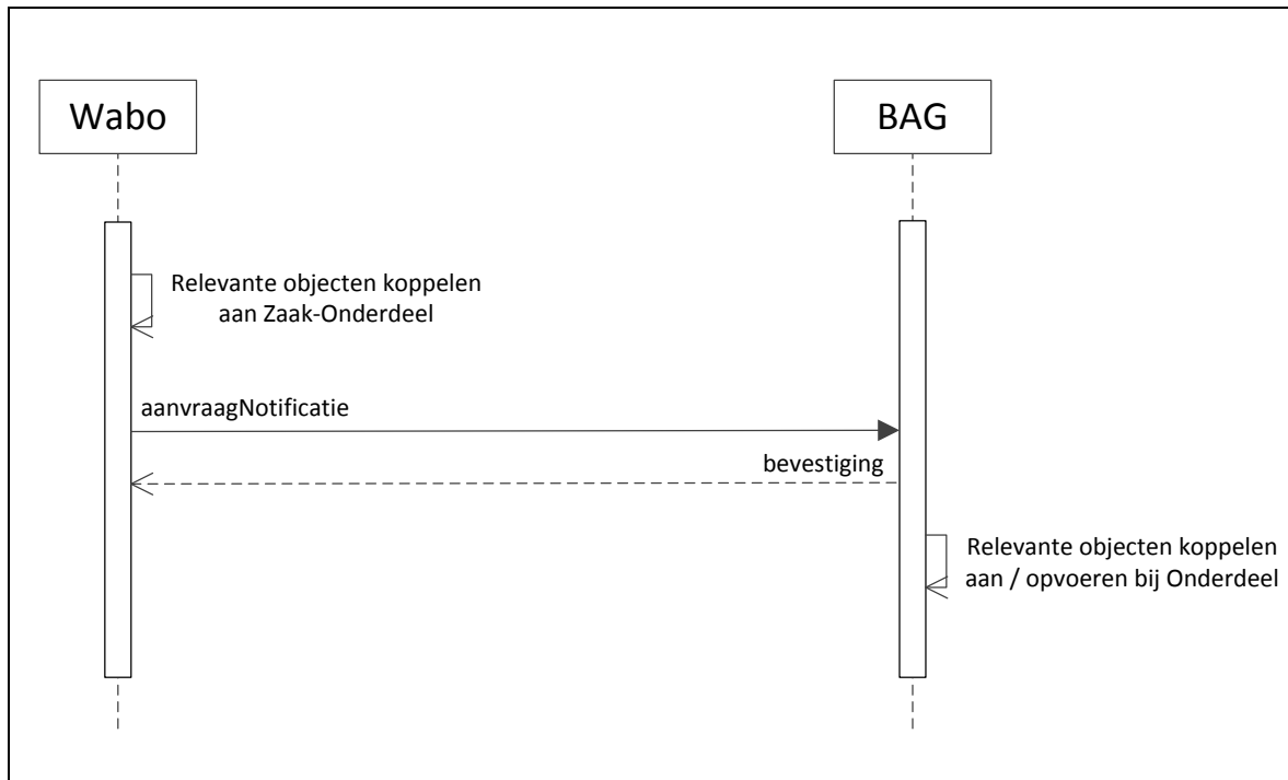
Figuur 6 Interactiemodel Aanvraagnotificatie
