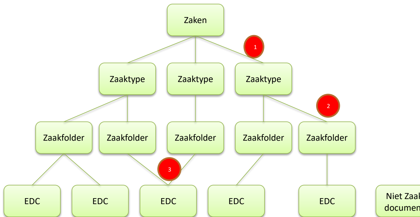
Figuur 26: Schematische weergave structuur van CMIS-repository
