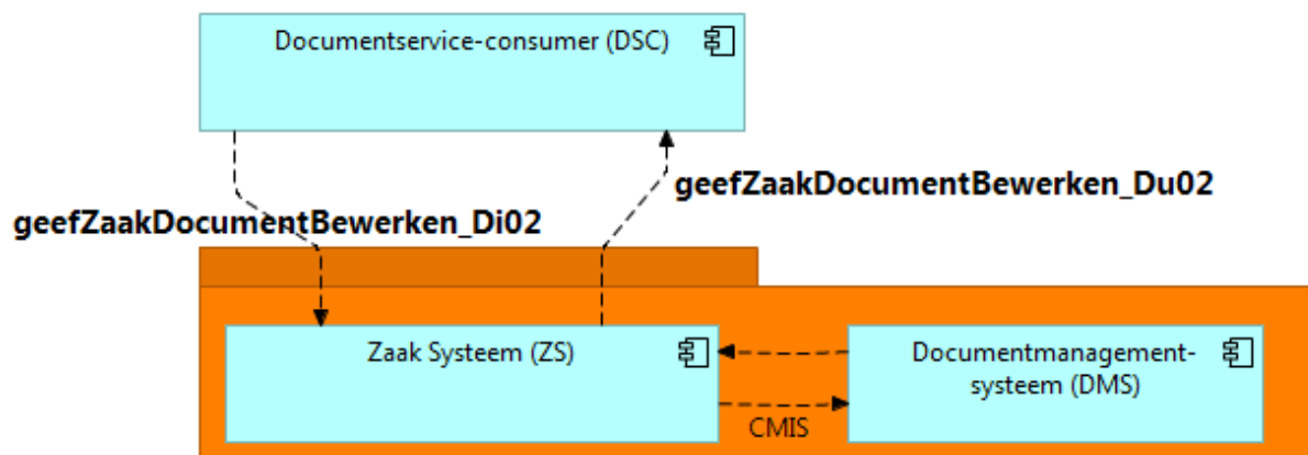
Figuur 19: Flow Geef Zaakdocument bewerken
